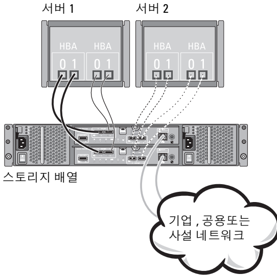
그림 2-4. 2 개의 컨트롤러에 연결된 2 개의 호스트
