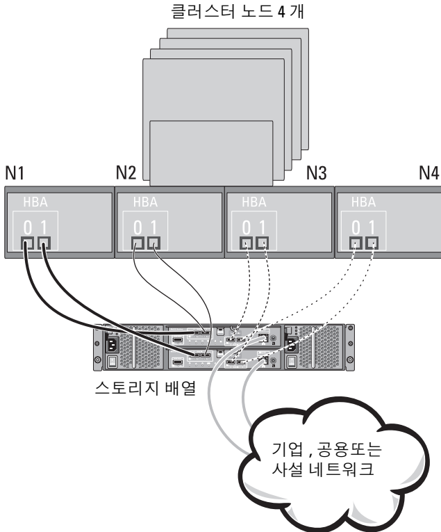
그림 2-8. 2 개의 컨트롤러에 연결된 4 개의 클러스터 노드
