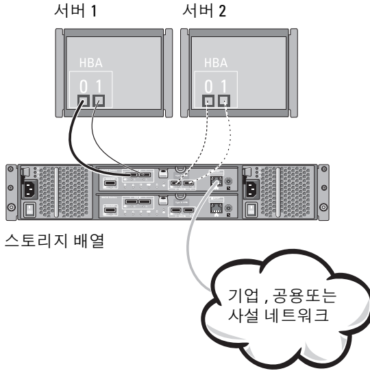
그림 2-2. 단일 컨트롤러에 연결된 2 개의 호스트
