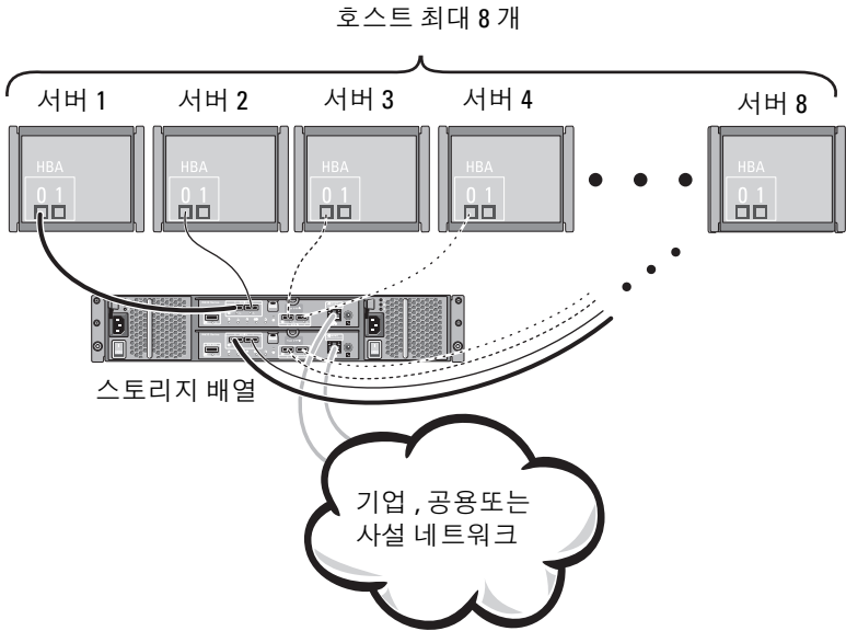
그림 2-7. 2 개의 컨트롤러에 연결된 8 개의 호스트
