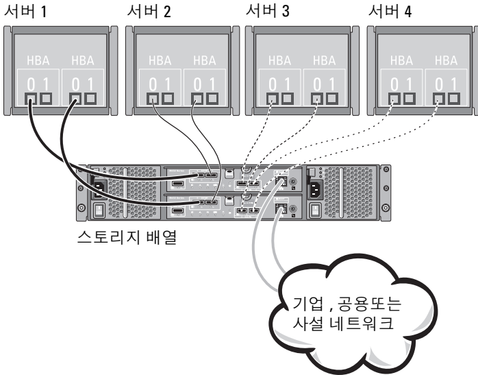
그림 2-5. 2 개의 컨트롤러에 연결된 4 개의 호스트
