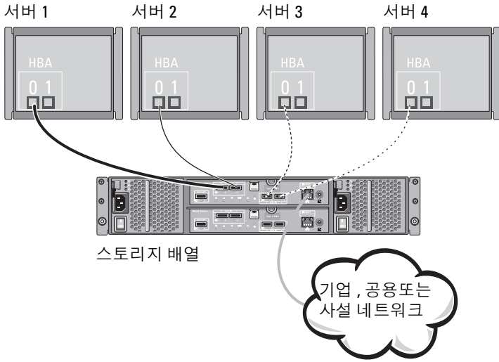
그림 2-3. 단일 컨트롤러에 연결된 4 개의 호스트
