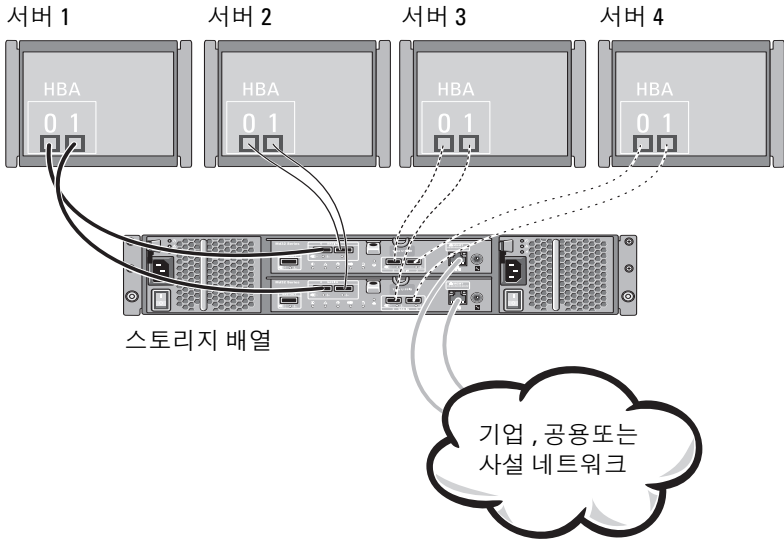
그림 2-6. 2 개의 컨트롤러에 연결된 4 개의 호스트
