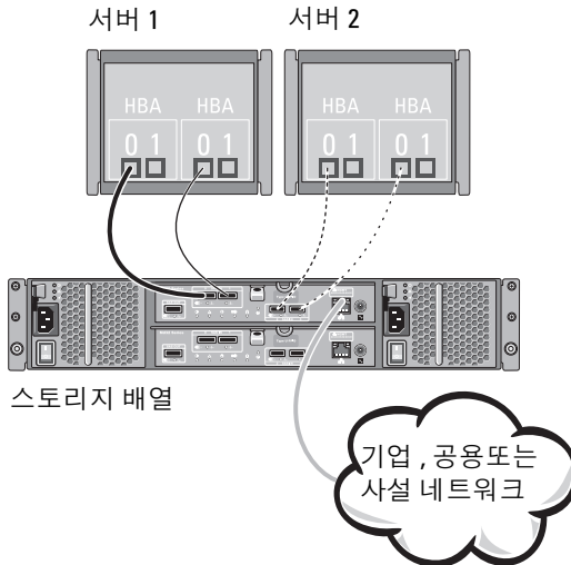
그림 2-1. 단일 컨트롤러에 연결된 2 개의 호스트
