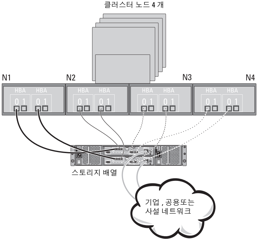
그림 2-9. 2 개의 컨트롤러에 연결된 4 개의 클러스터 노드
